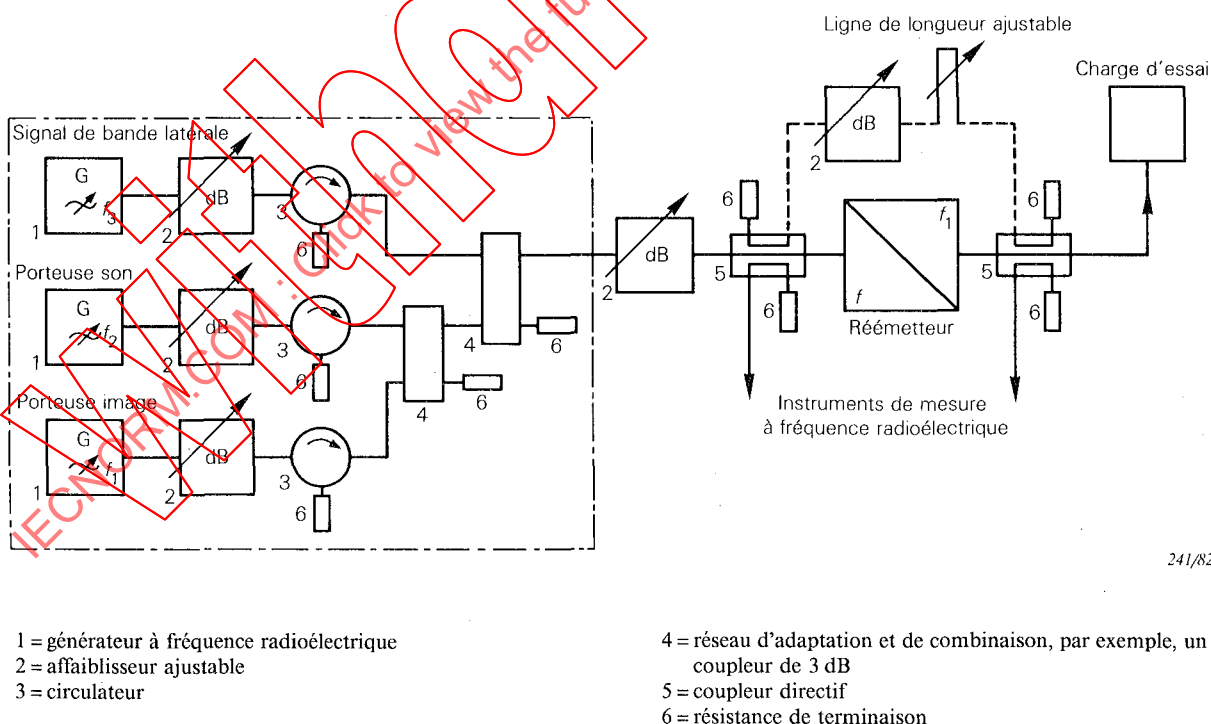
FIG. 1. — Exemple de dispositif A utilisant trois générateurs à fréquence radioélectrique.
