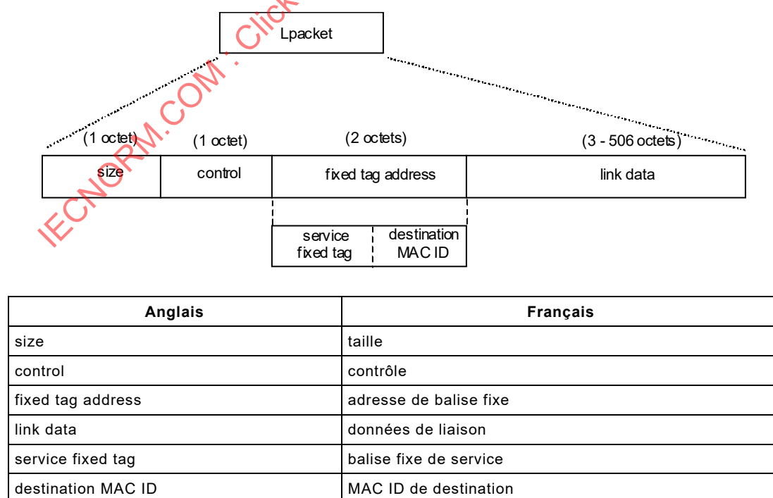
Figure 14 – Format Lpacket à balise fixe
