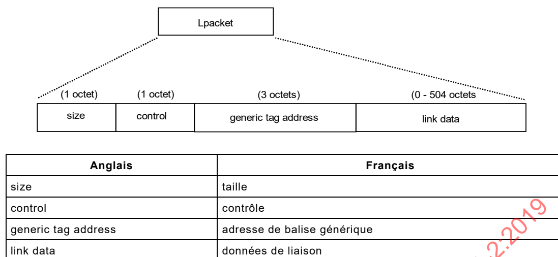
Figure 13 – Format Lpacket à balise générique
