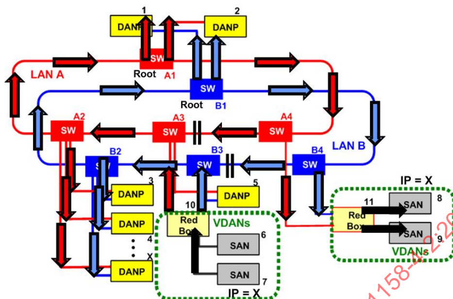
Figure 45 – Virtual DANs
