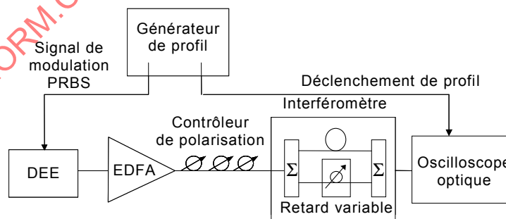
Figure 7 – Montage de la méthode du discriminateur en fréquence
