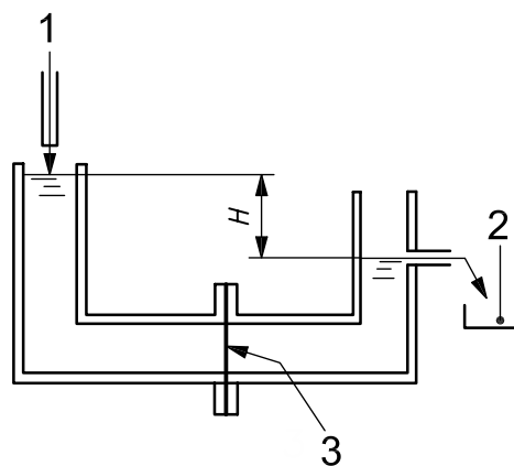
a) Horizontal
