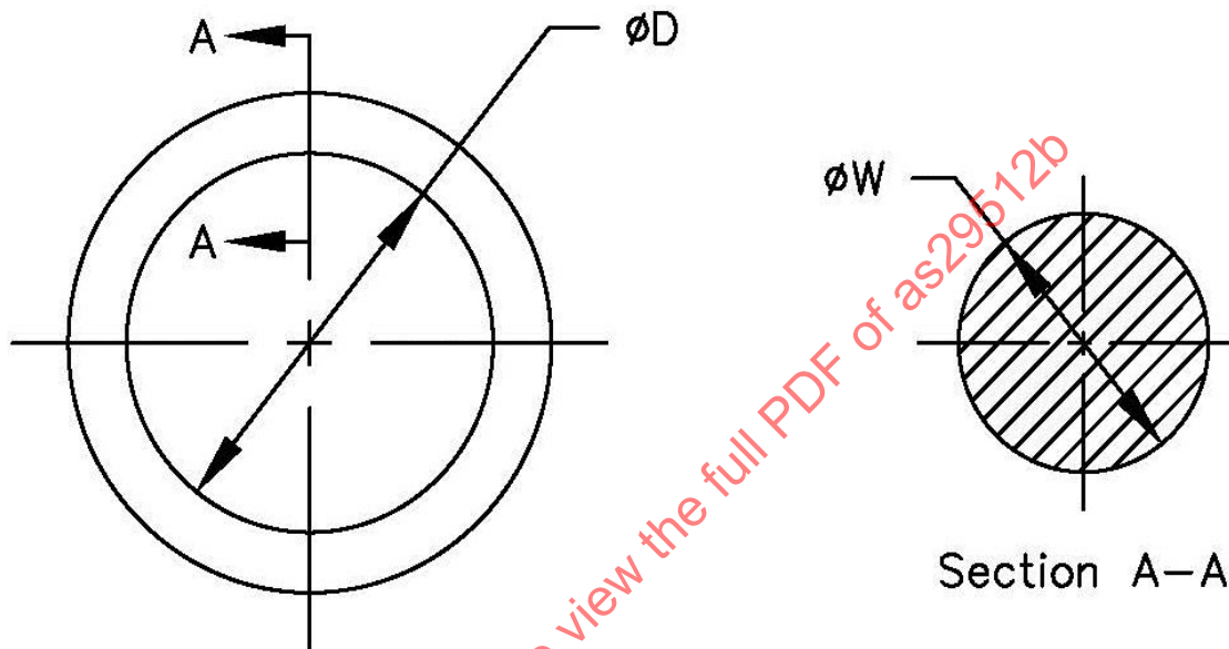
FIGURE 1 - O-RING: WIDTH (W) AND INSIDE (D) DIAMETERS
